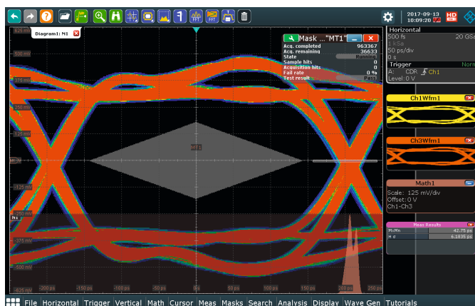
Преимущества быстрого тестирования по маске и отображения гистограммы
