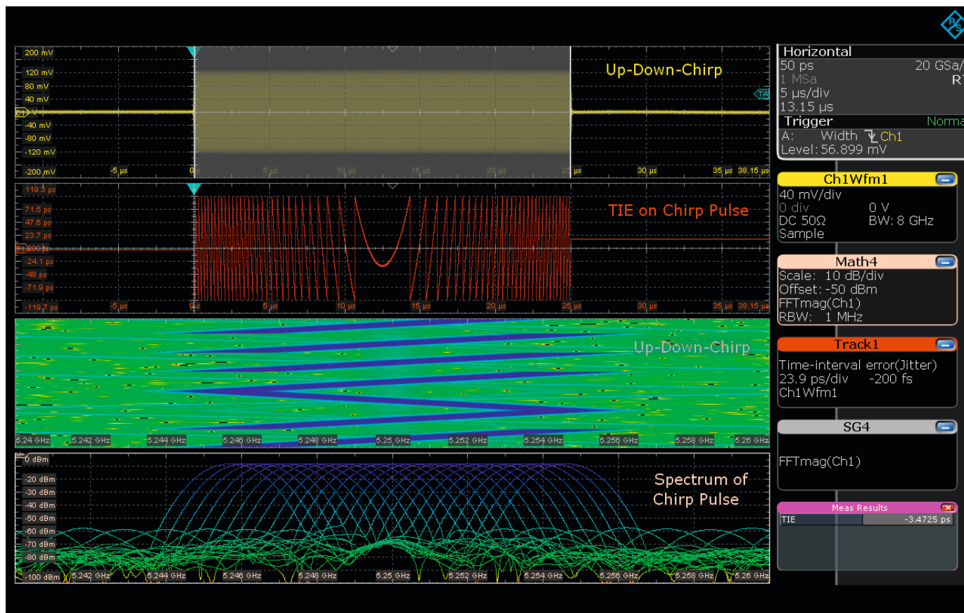
Импульсный анализ ЛЧМ-сигнала во временной и частотной областях
