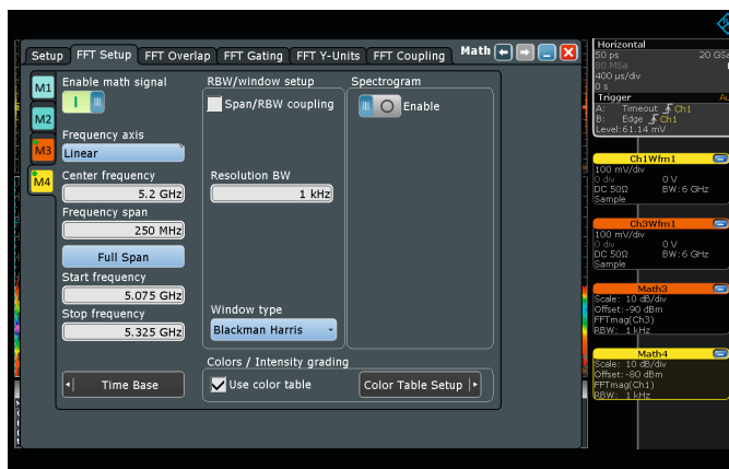
Настройка частотного анализа упростилась с помощью типовых параметров
