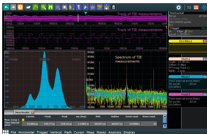
Обнаружение частотных помех в тактовом сигнале: отслеживание TIE-джиттера; гистограмма и БПФ-анализ кривой трека
