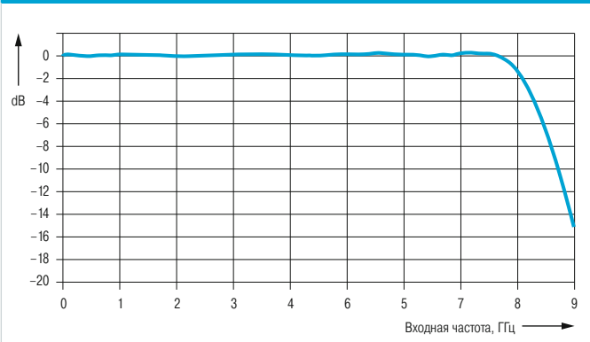
Плоская частотная характеристика осциллографа R&S®RTP084
